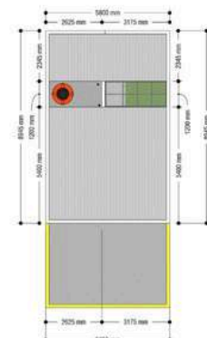
Layout Rencana Atap
